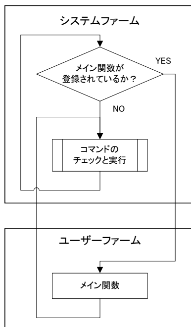
図 5 自律動作
