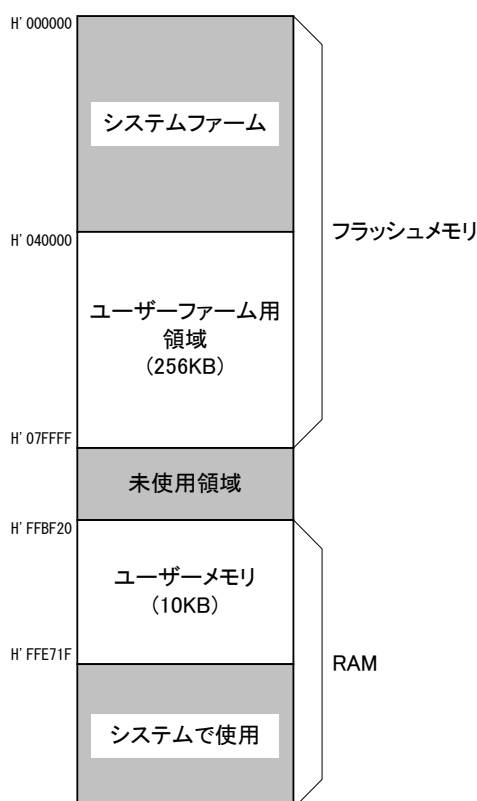
図 6 メモリ空間
