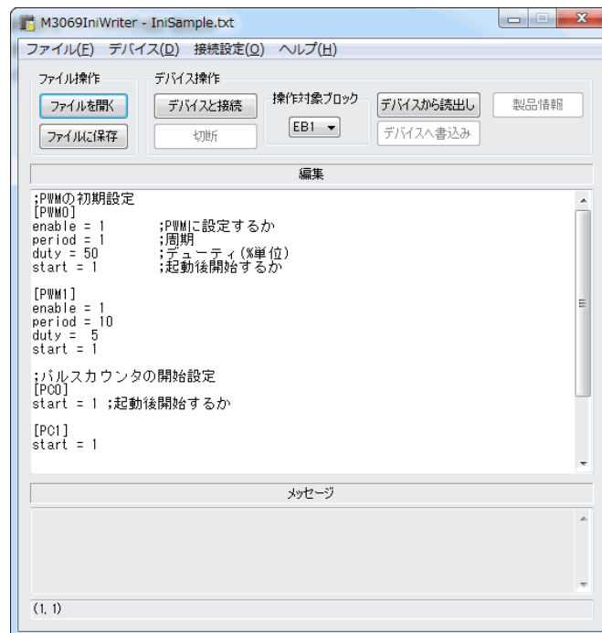
図 53 「M3069IniWriter」の画面
