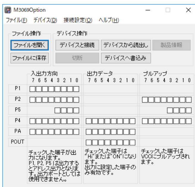
図 11 「M3069Option」の画面
