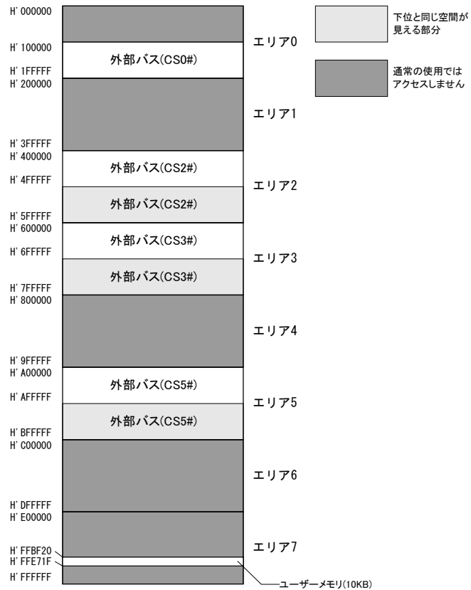
図 6 メモリマップ
