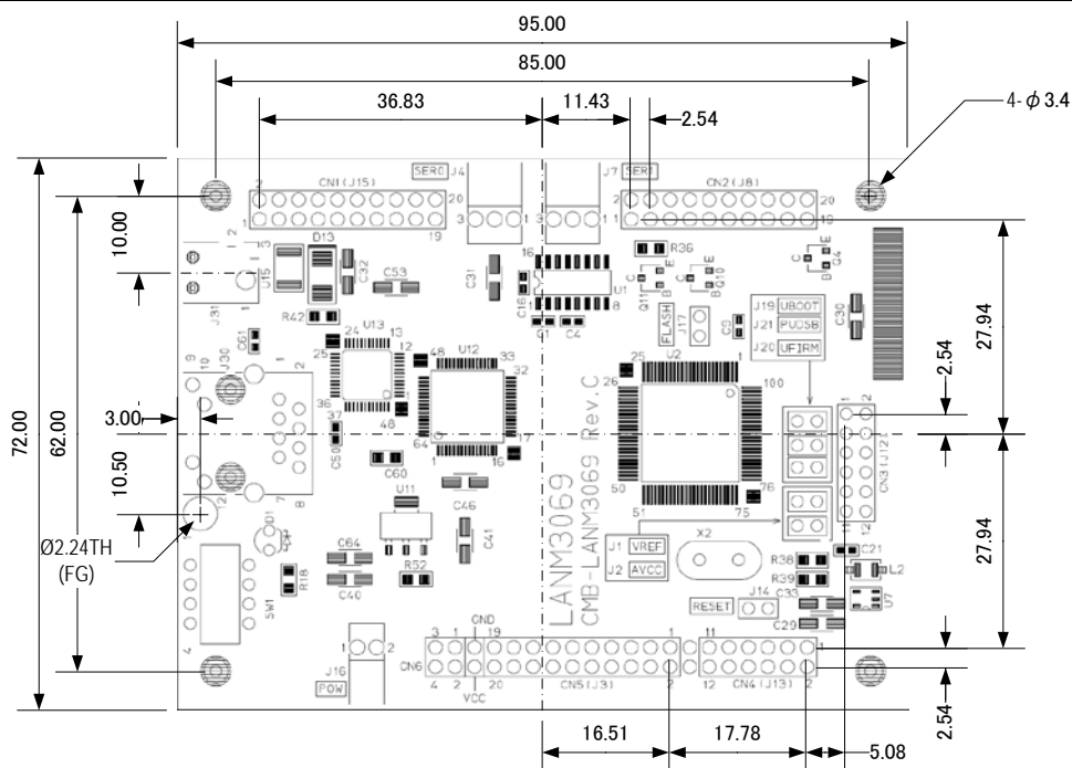
図 3 基板図
