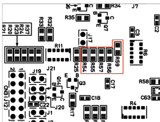
図 14 変更部品位置 (半田面)
