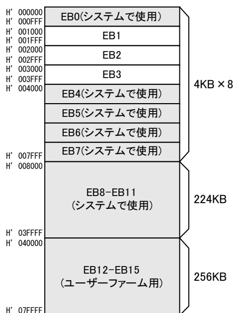
図 7 フラッシュメモリマップ
