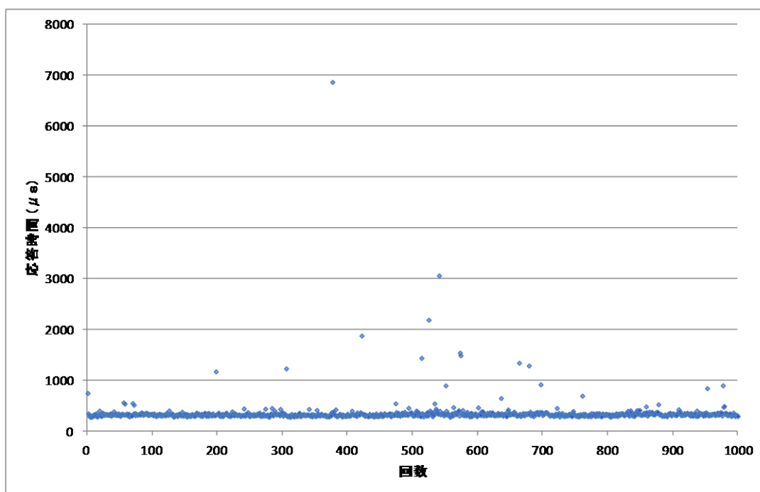
図 13 製品の応答時間
