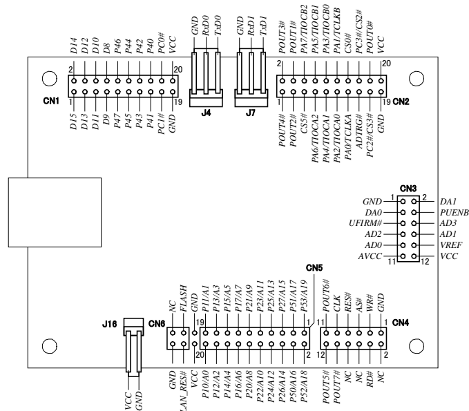
図 4 信号配置図
