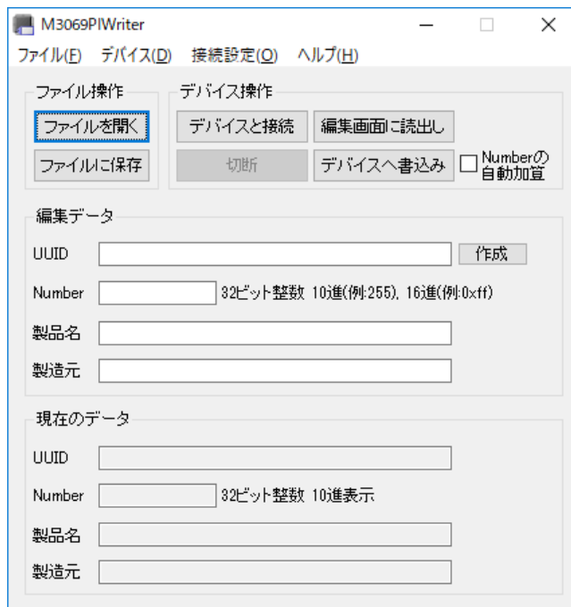
図 9 「M3069PIWriter」の画面
