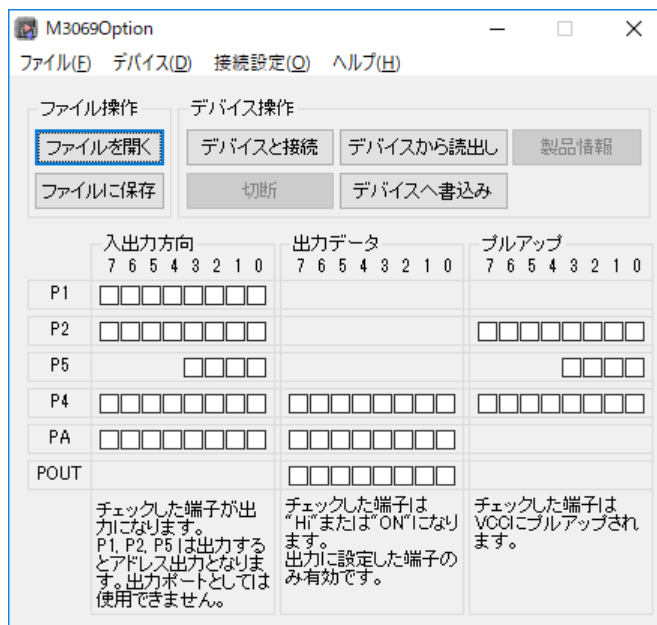
図 10 「M3069Option」の画面
