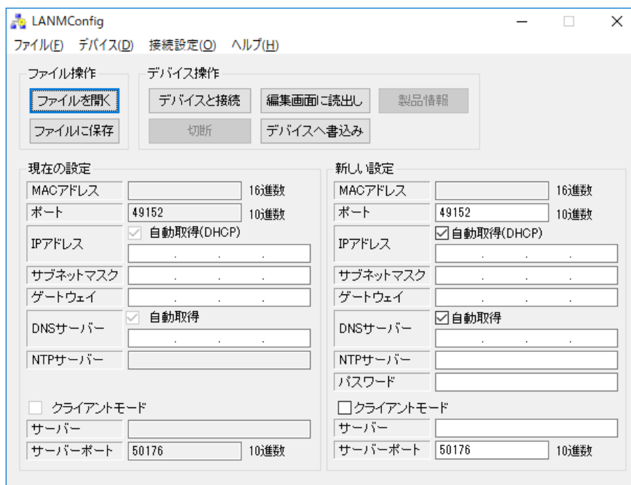
図 8 「LANMConfig」の画面
