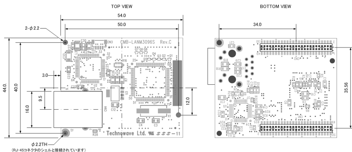
図 4 基板図
